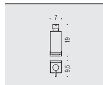
B9316 Spandisapone (L 0,31) Distributeur à savon
